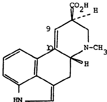
lysergic acid (2)-aΔ 9,10 -ergolene
