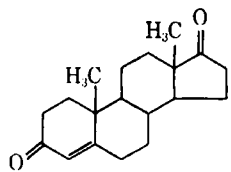
VIII: 4-androstene-3,17-dione
