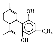
II: cannabidiol
