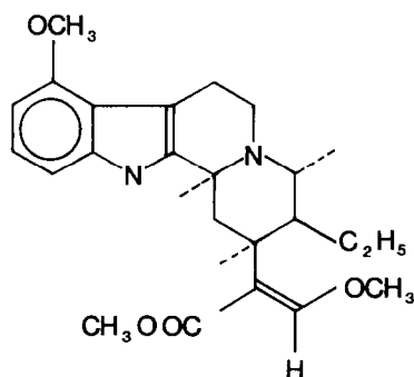
Fig. 1. Mitragynine.
