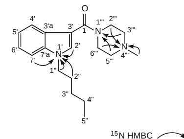
(d) Compound (2)
