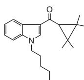
UR-144
