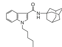
APICA
