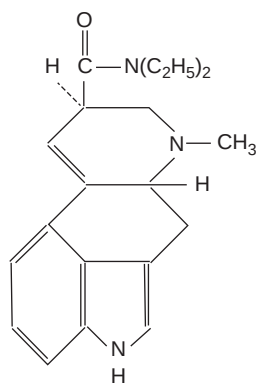
LSD-25
