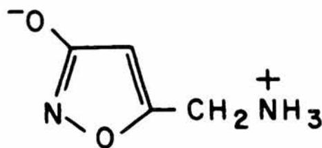
MUSCIMOL
