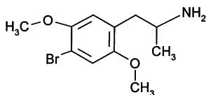
2-CB (4-bromo-2,5-dimethoxyphenylethylamine)
