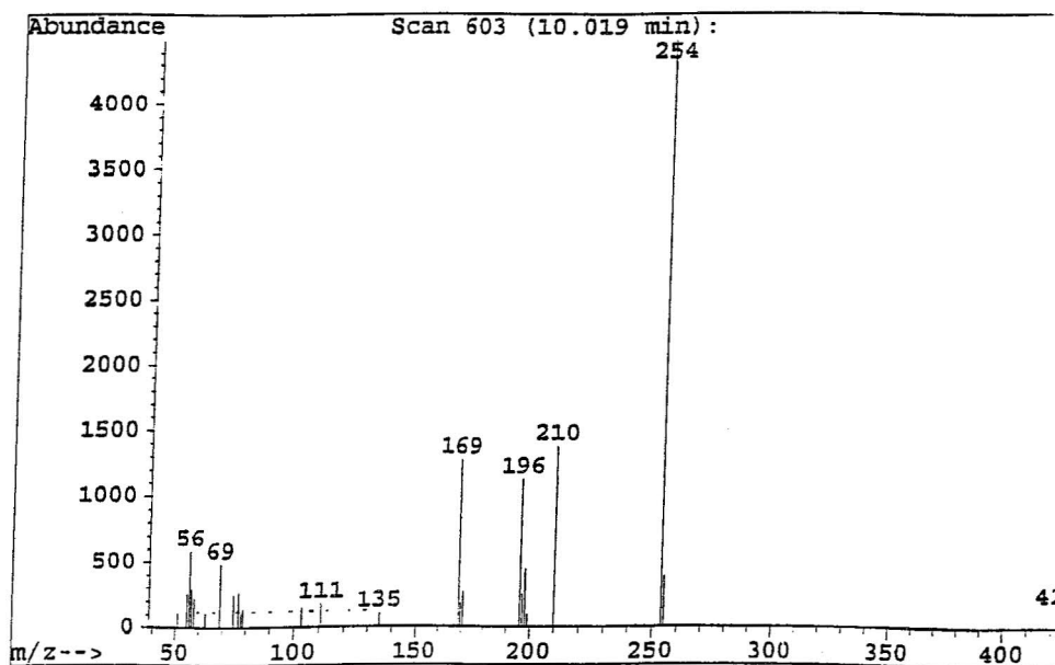
FIG. 2b—EI/MS of Cl-MDMA.
